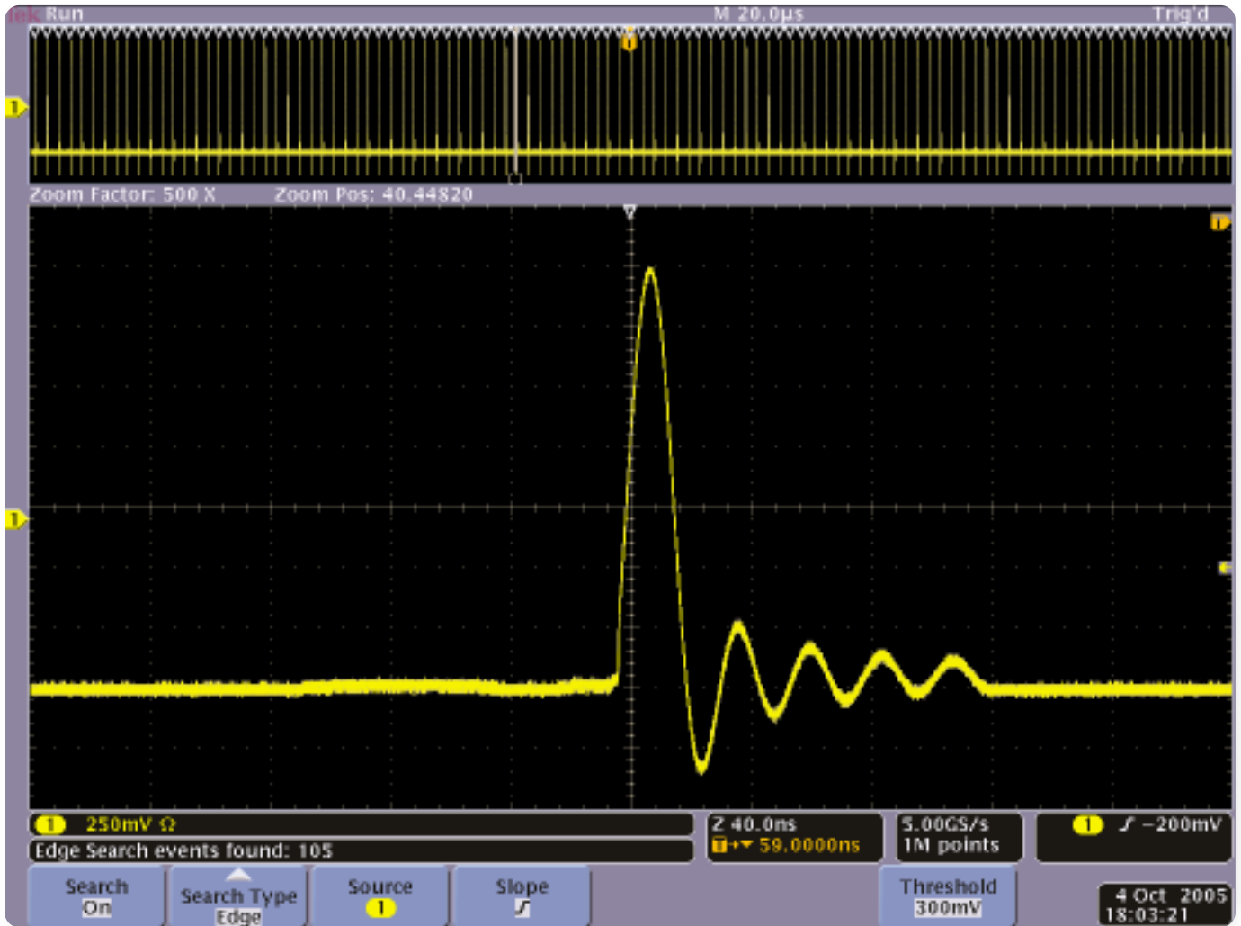
▶ 그림 4. DPO4000 시리즈는 긴 획득 데이터에서 300mV를 통과하는 모든 펄스를 표시합니다.
