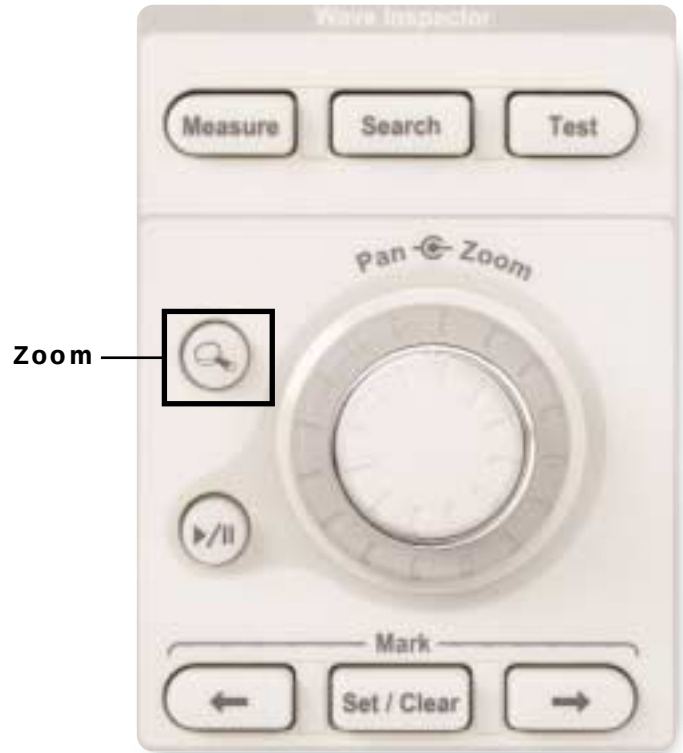
▶ 그림 1A. Wave Inspector에는 전용 전면 패널 확대/축소 (zoom) 및 팬(pan) 컨트롤이 있습니다.
