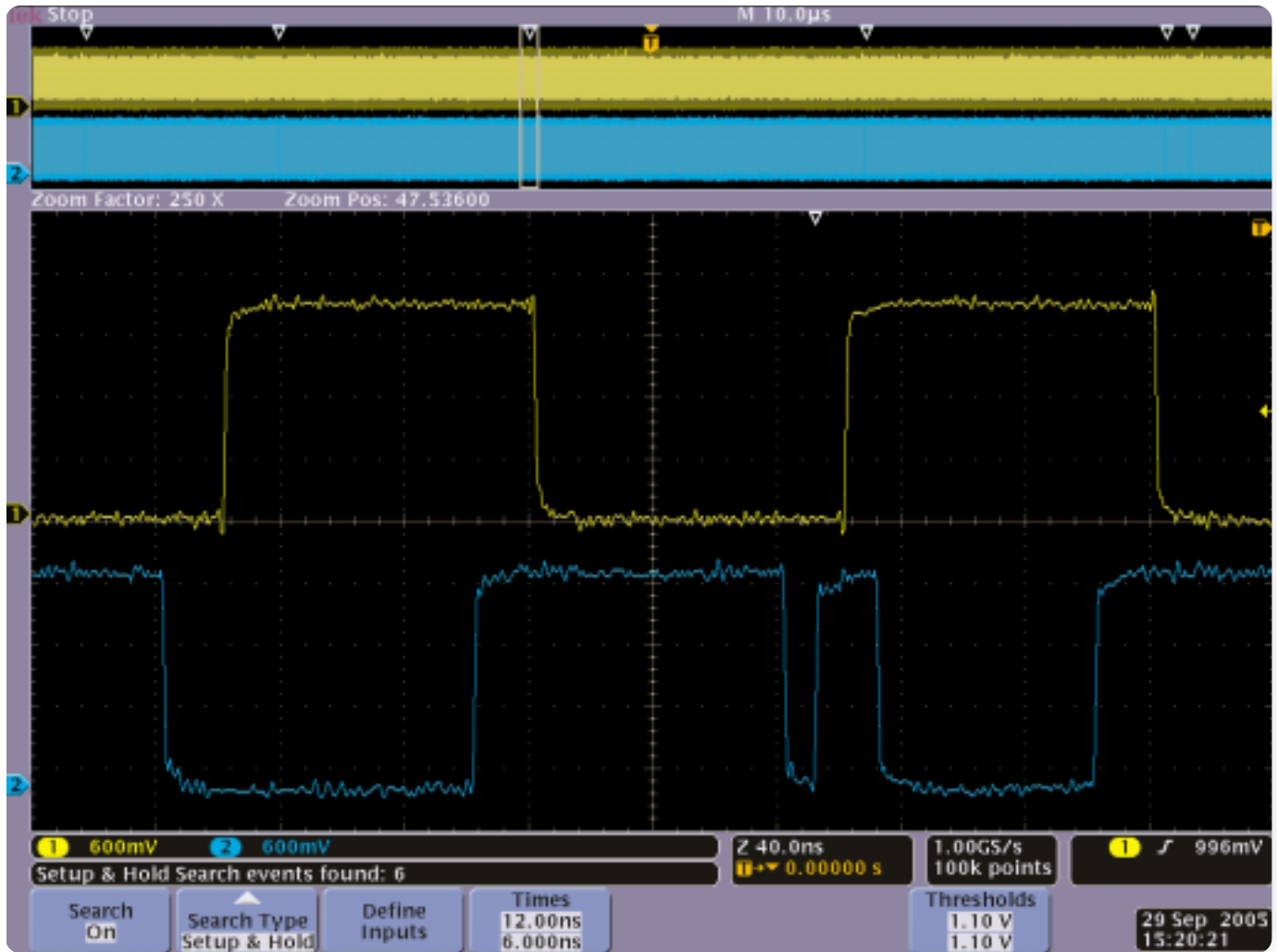
▶ 그림 5. 셋업 및 홀드(Setup & Hold) 위반 검색을 통해 6개의 위반 이벤트가 발견되었습니다
