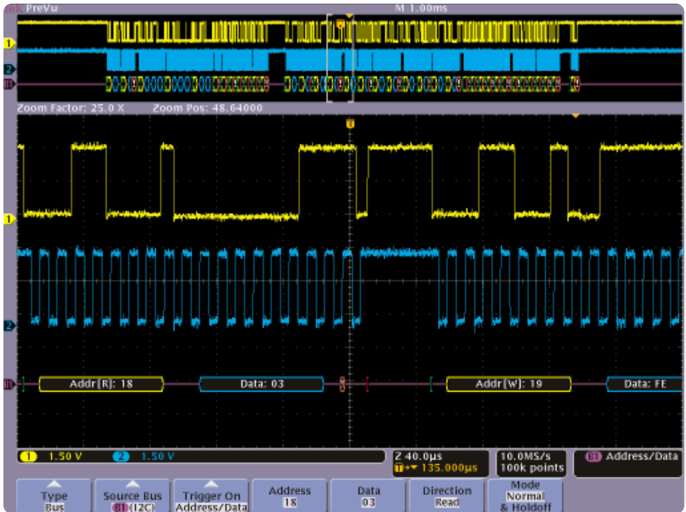
▶ 그림 2. I 2 C 버스의 긴 획득을 통해 이동
